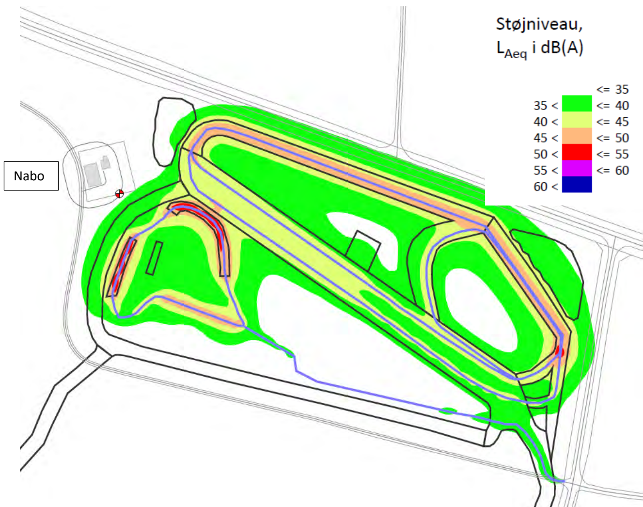
Figur 7.3: Illustration af støjudbredelsen fra Manøvrebanelen.
