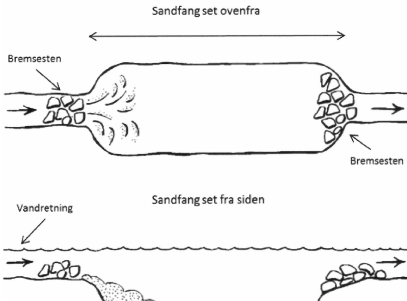
Principskitse af sandfangets form med udlæg af sten ved ind- og udløb.
