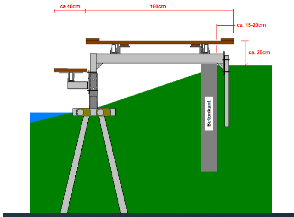
Tegning over platform langs Freerslev Å.
