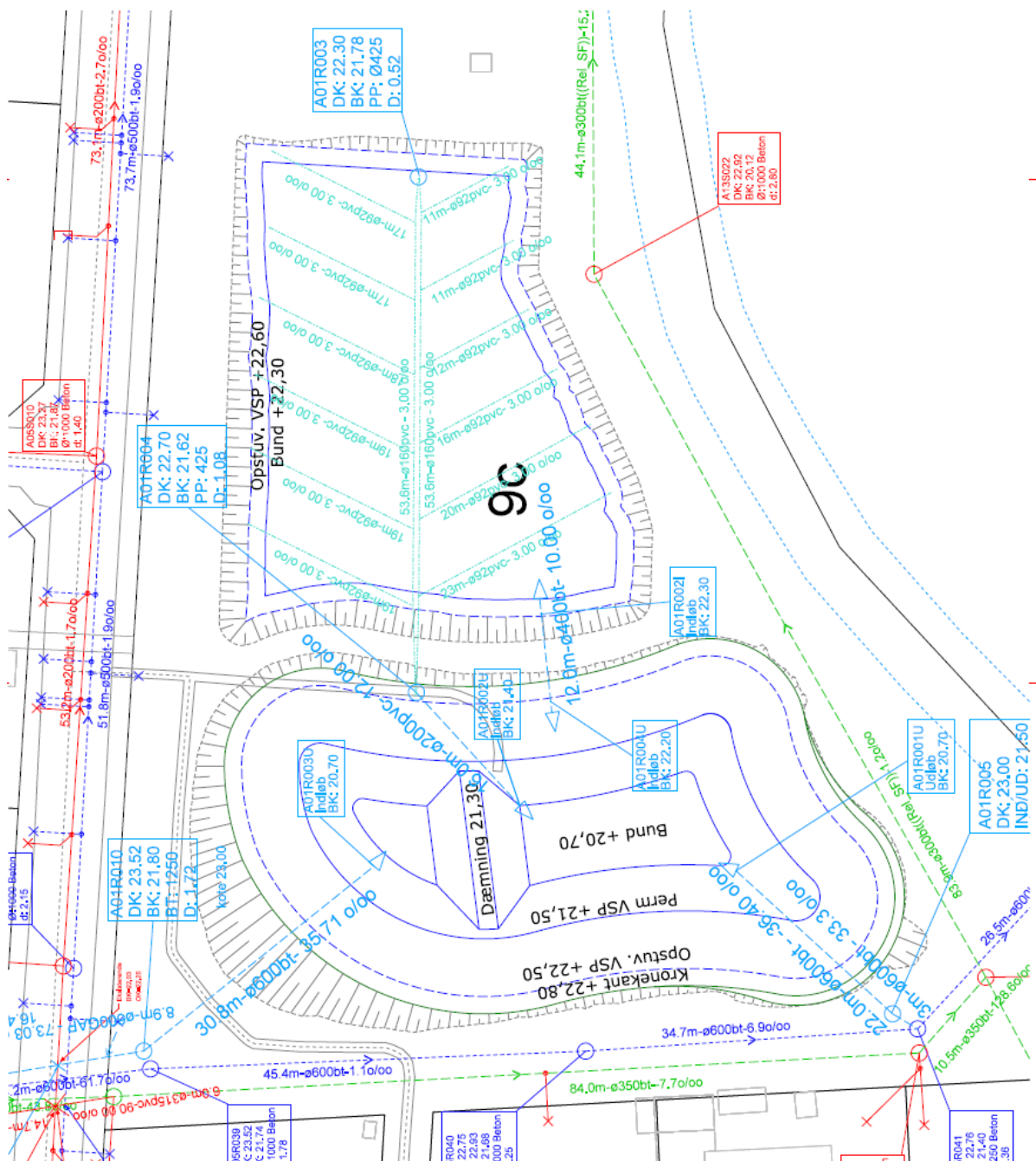
Kort 4 – Udklip af den tekniske tegning over regnvandsbassinerne, der viser placering af rør, dræn mm.
