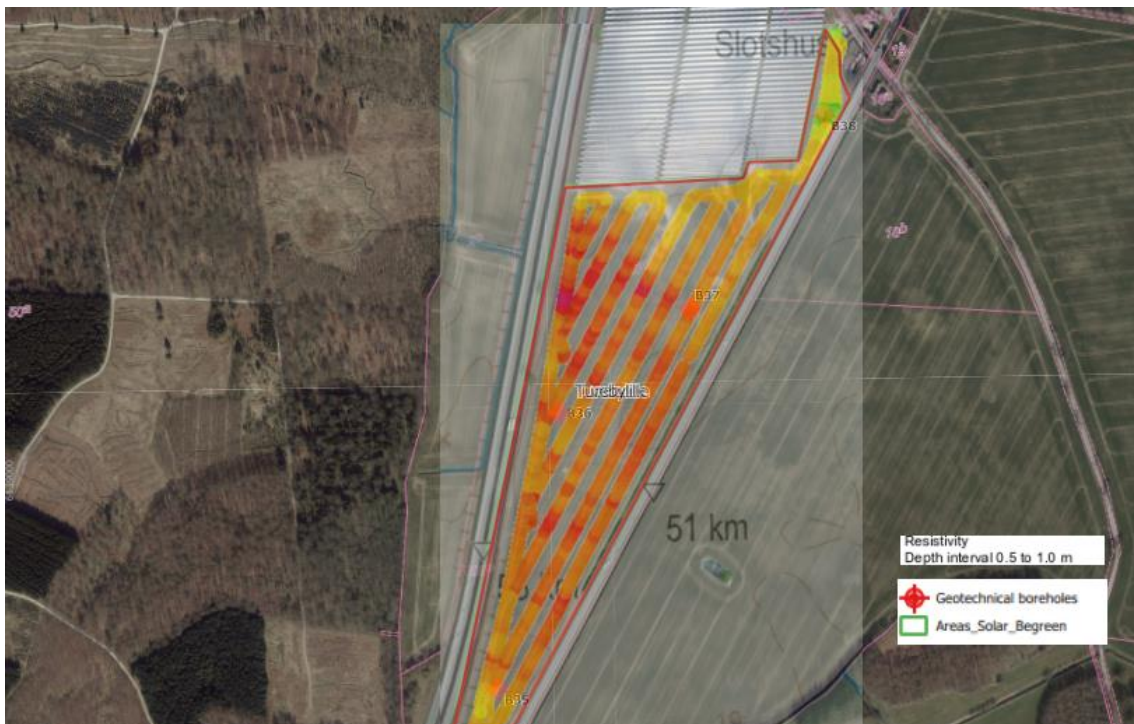
Figur 4. Kortet viser placeringerne af de geotekniske borer og resultaterne af den fladedækkende geofysiske undersøgelse med DualEM. Lilla og røde farver indikerer overvejende sandede aflejringer, mens blå og grønne farver indikerer mere finkornede aflejringer som silt, ler og tørv/gytje.
