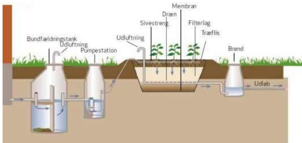
Figur 6. Beplantet filteranlæg.
