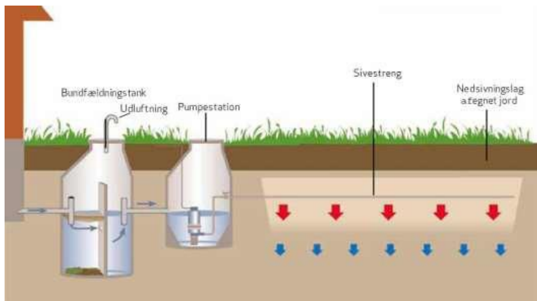
Figur 2. Nedsivningsanlæg.
