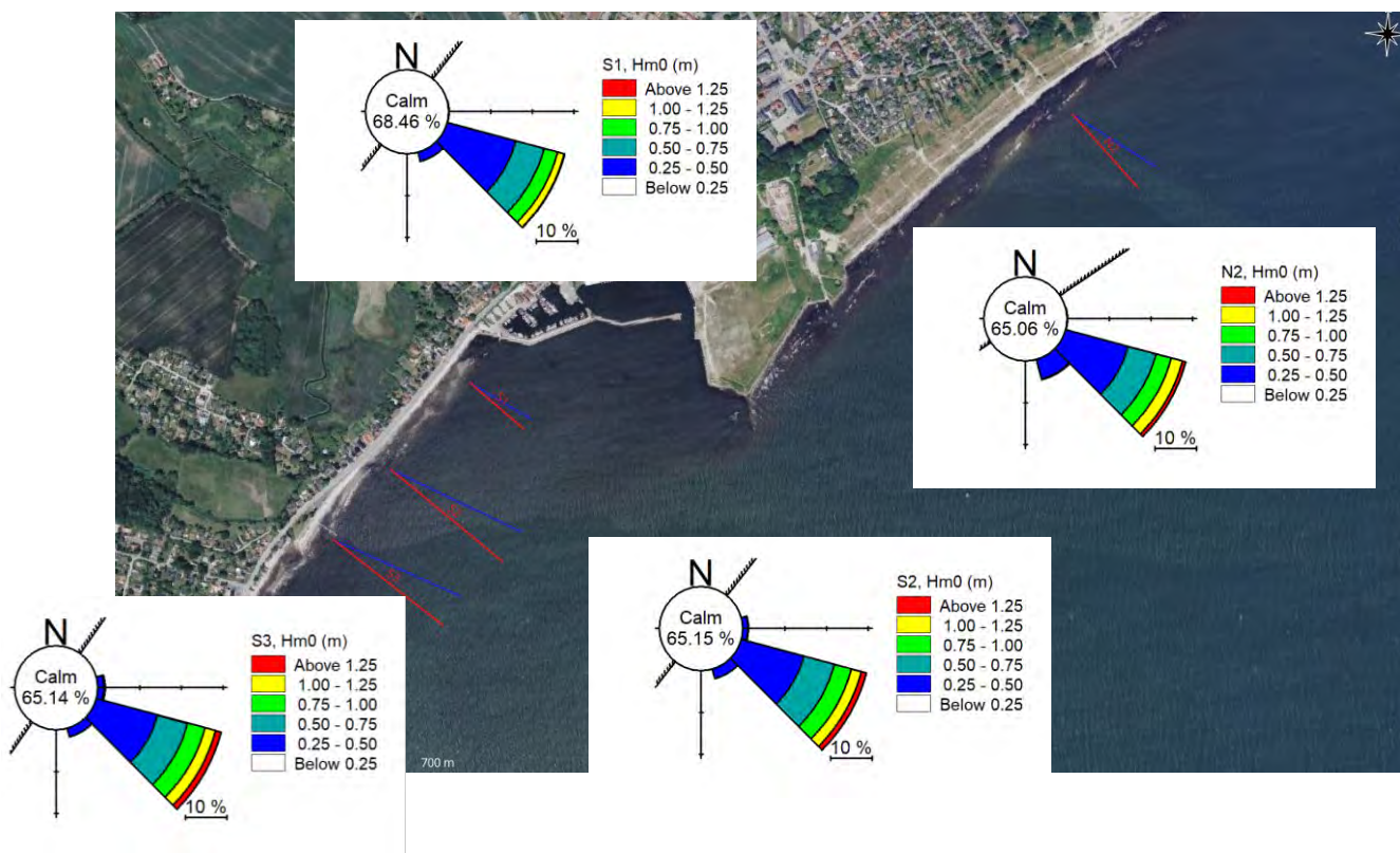
Figur 4.5 Bølgeroser for bølgeforcing anvendt til Litdrift modellering af eksisterende forhold.
