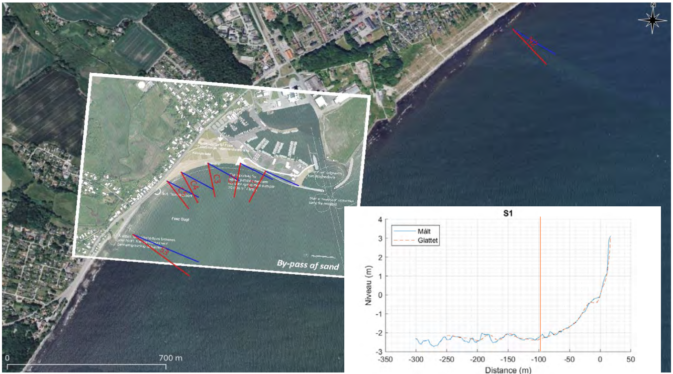
Figur 4.6 Profilver og batymetri for fremtidige forhold langs Sydstranden.
