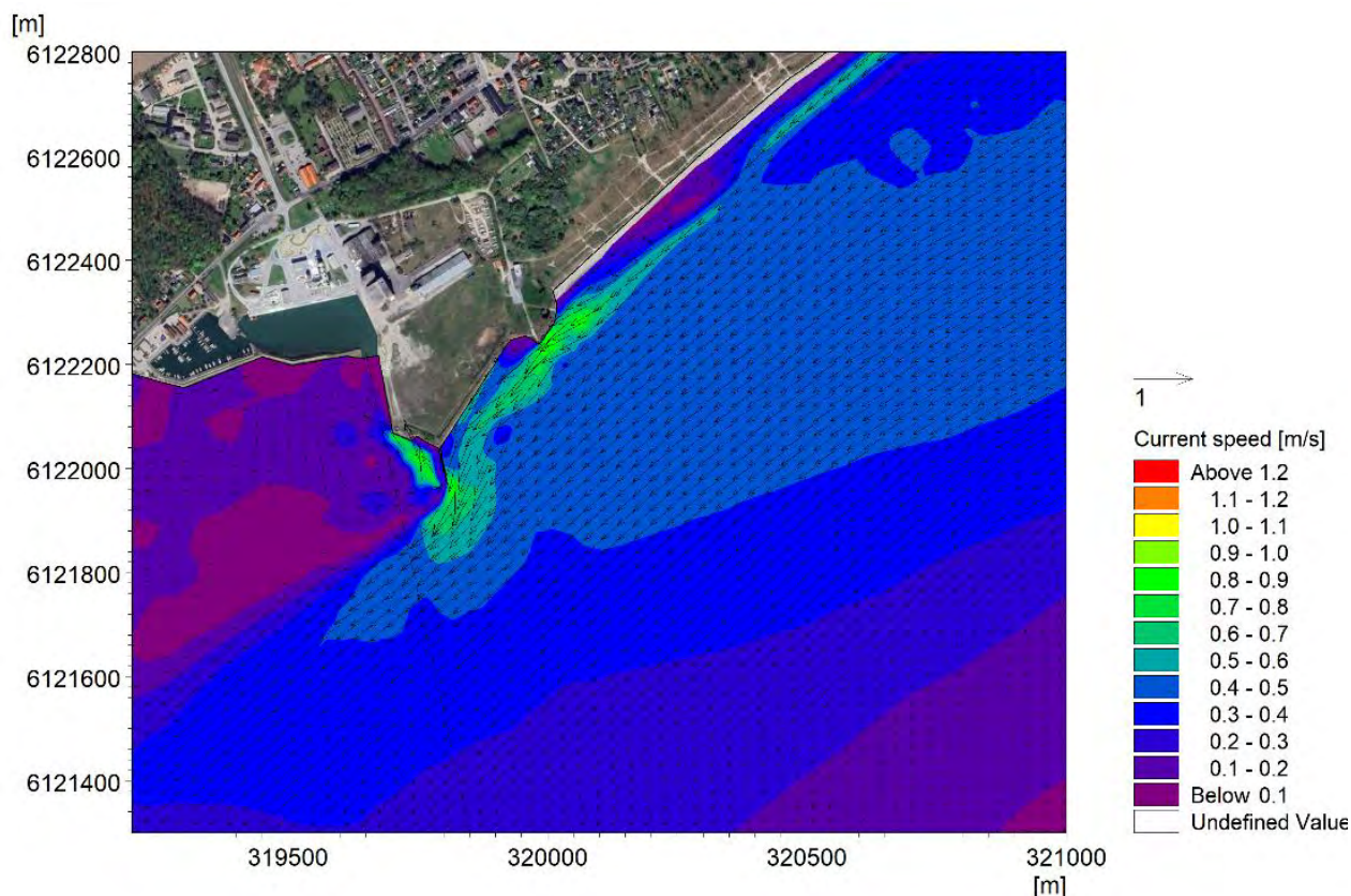
Figur 7.1 Kort, der viser strømforholdene omkring den eksisterende havn under en kraftig stormhændelse. Bølgeforholdene på modellens rand er i dette scenarie H_s = 2 m, T_p = 7 s og MWD = 90^\circ .
