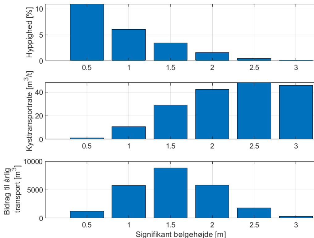
Figur 6.7 Søjlediagrammer, der illustrerer hyppighed og transport for de betragtede bølgescenarier.
