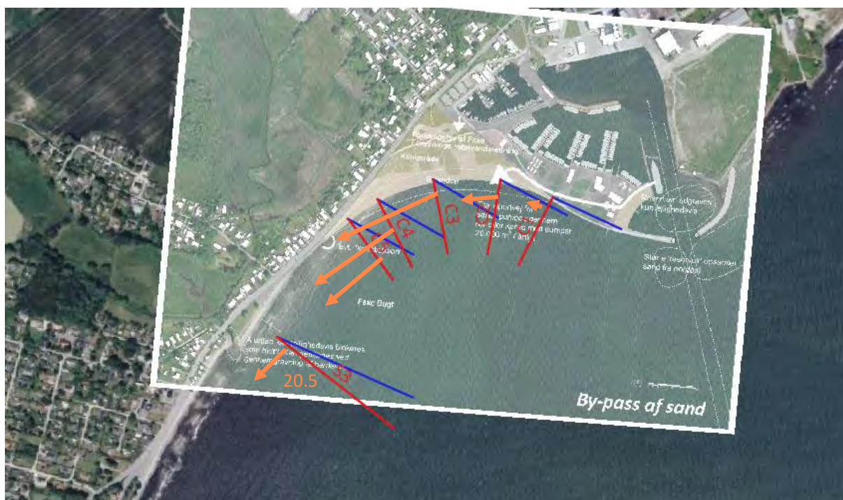
Figur 5.7 Oversigtskort for modelleret kysttransport (orange pile) under fremtidige forhold. Røde profiler angiver kystens målte orientering baseret på Google Earth. Blå profiler markerer den beregnede klassiske ligevægtsorientering.
