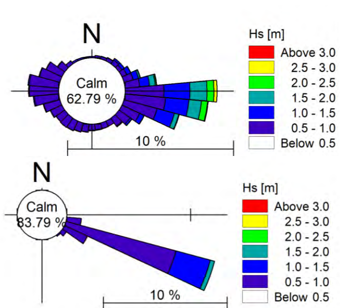
Figur 5.2 Bølgeroser, der viser bølgeklimate i midten af Faxø Bugt (øverst) og tæt på Faxø Ladeplads Havn (nederst).
