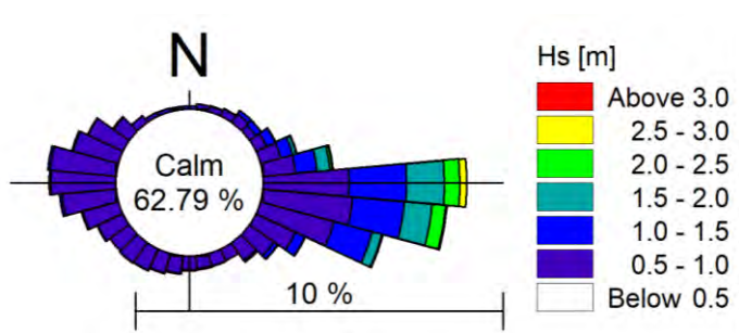
Figur 3.5 Bølgerose, der viser bølgeforhold i Faxe Bugt.
